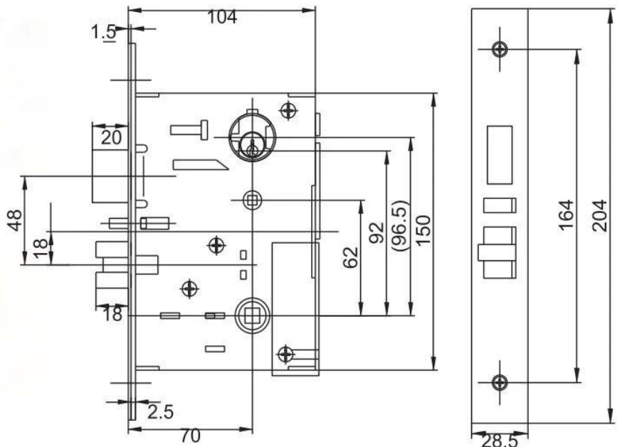
Mortise ANSI
